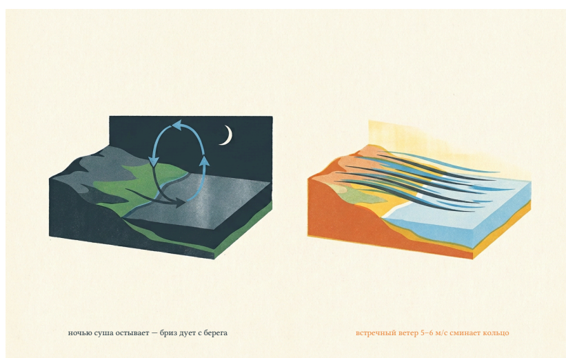
Рис. 2. Ночью циркуляция переворачивается: остывшая суша холоднее воды, и бриз дует с берега. При фоновом ветре 5–6 м/с кольцо не складывается вовсе. Схема.
