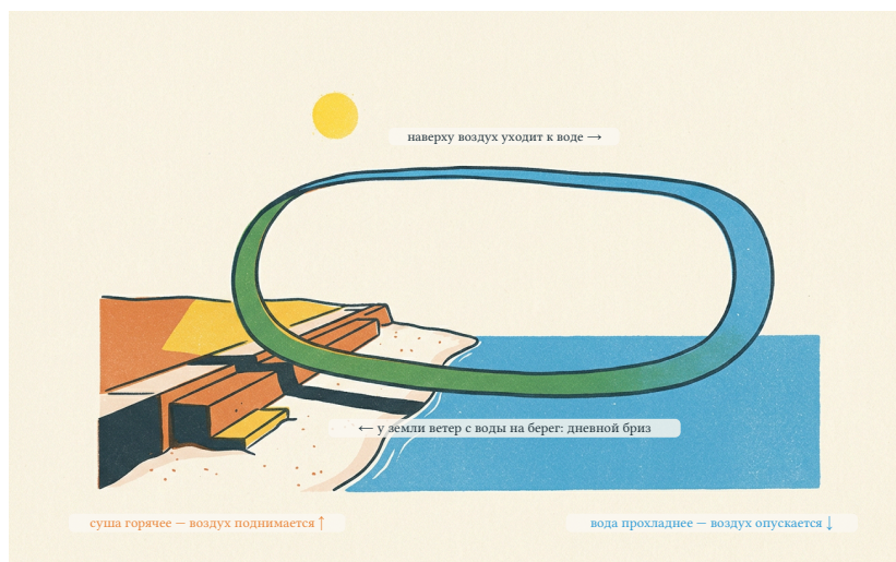
Рис. 1. Кольцо дневного бриза: воздух над горячим берегом поднимается, над прохладной водой опускается, а приземную ветвь этого кольца мы и чувствуем как ветер с воды. Схема.
