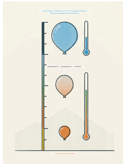
Рис. 1. Поднимающийся воздух остывает сам, без подвода холода: расширяясь, он тратит энергию. Сухой — почти ровно на 9,8 градуса на километр. Схема.
