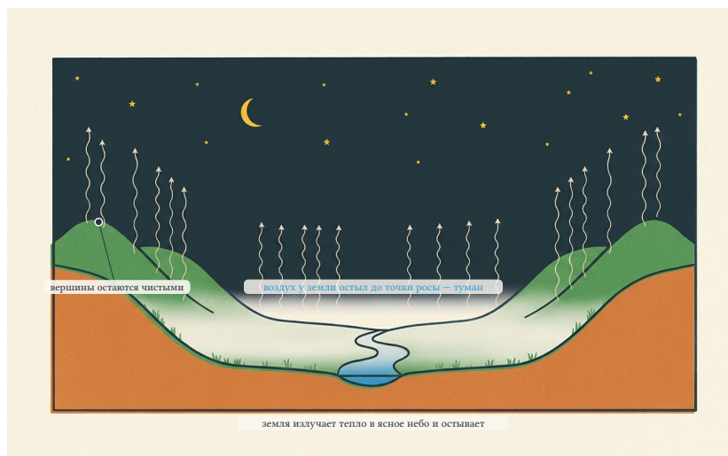
Рис. 2. Радиационный туман: ясной ночью земля остывает, охлаждает прилегающий воздух, и пар в нём достигает насыщения. Туман растёт от земли вверх. Схема.
